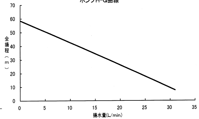
ポンプH-Q曲線
