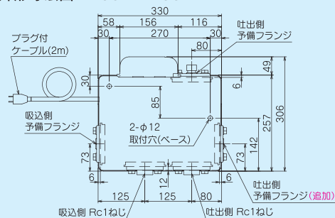
■外形寸法図 150W~250W
