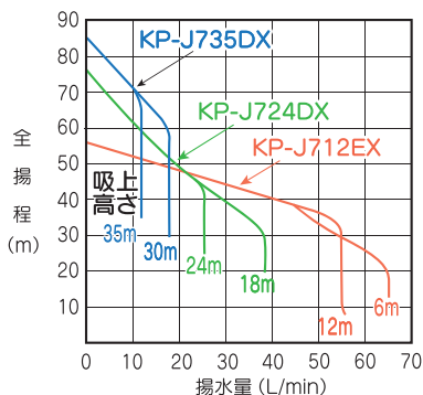
■選定図 KP-3755LT-1/3756LT-1
