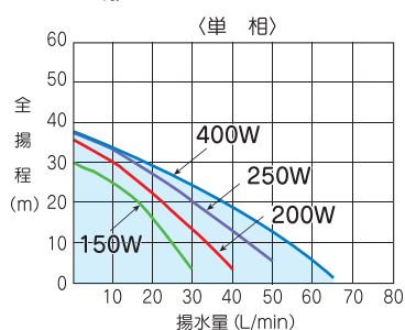
THP6形 ■選定図 (50Hz,60Hz 共通)
