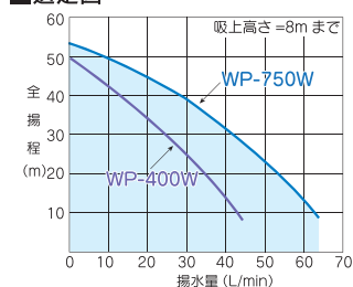
■選定図
