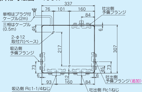
■外形寸法図 400W
