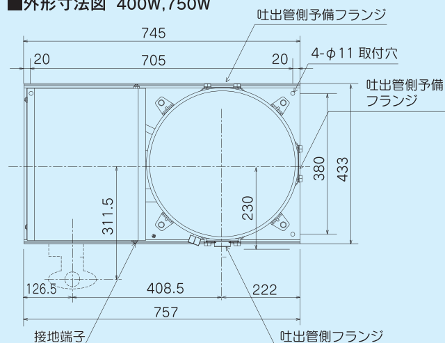
■外形寸法図 400W,750W
