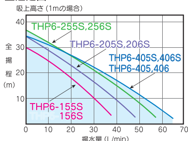
■選定図
