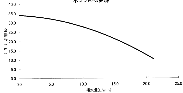
ポンプH-Q曲線
