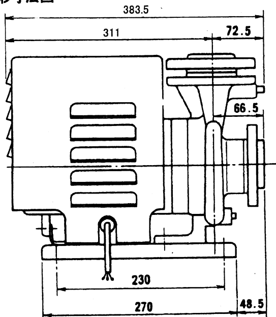
外形寸法図
