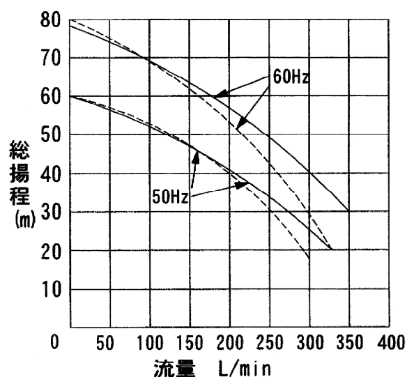
ポンプ特性
