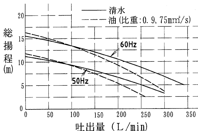
ポンプ特性
