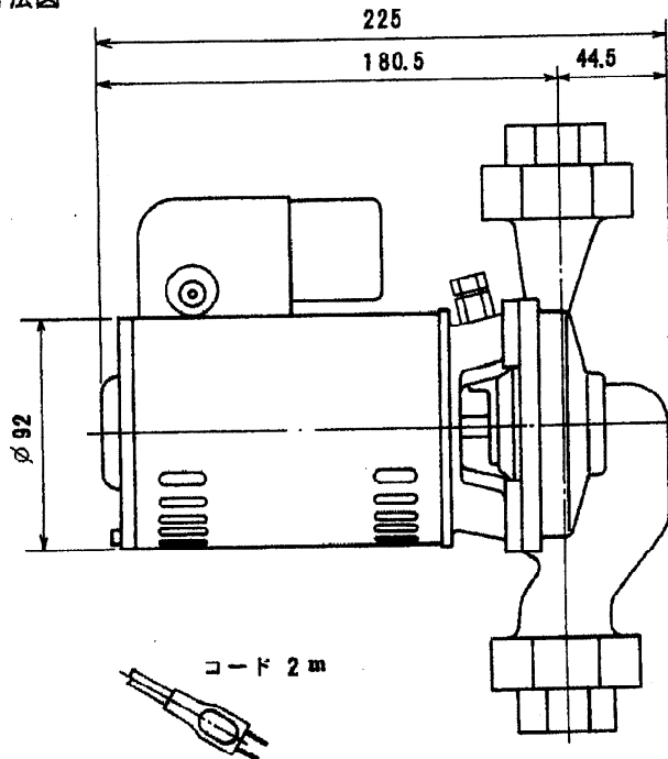
外形寸法図
