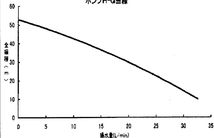
ポンプH-Q曲線
