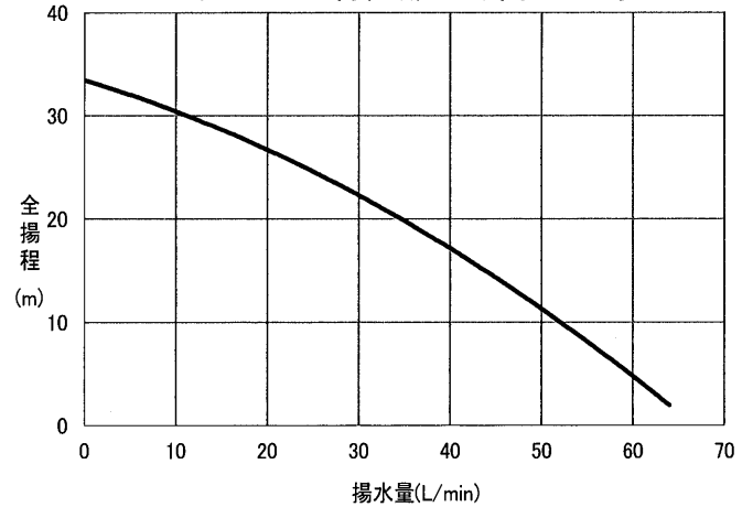
ポンプH-Q特性(吸上げ高さ1m時)
