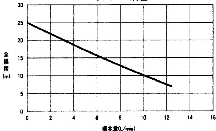
ポンプH-Q特性
