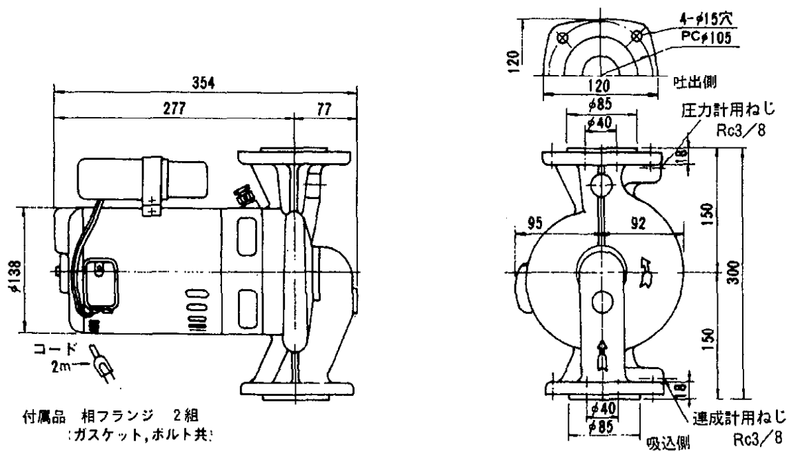
外形寸法図
