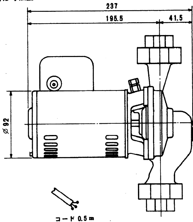
外形寸法図
