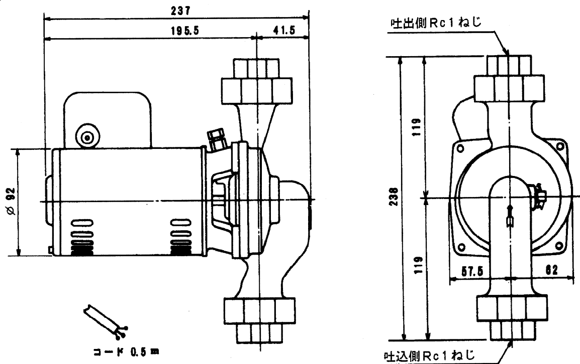
外形寸法図
