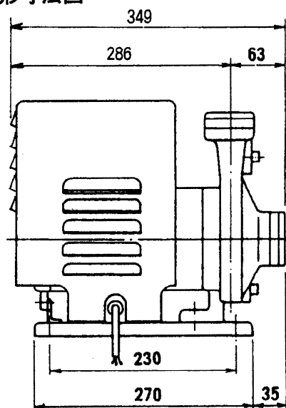
外形寸法図
