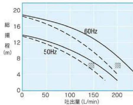
NQJ-700E・NQJ-e750
