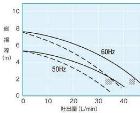
NQJ-60E
