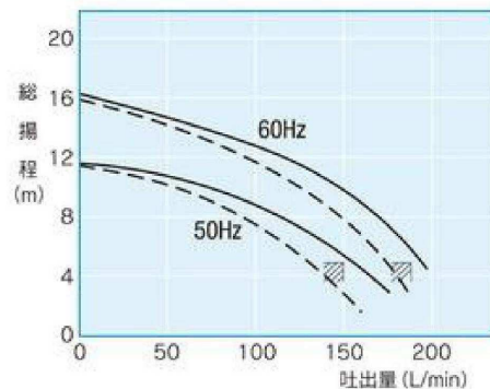
NQJ-400E, NQJ-S400E-180
