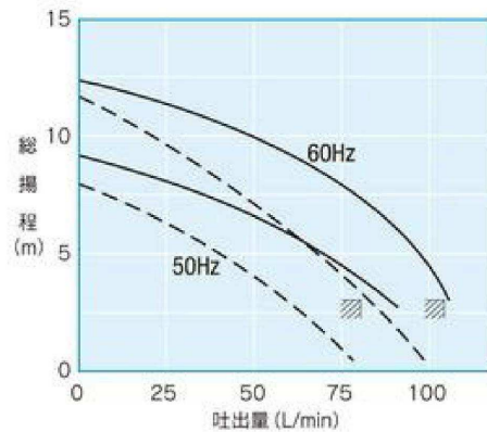
NQJ-180E, NQJ-S180E-240
