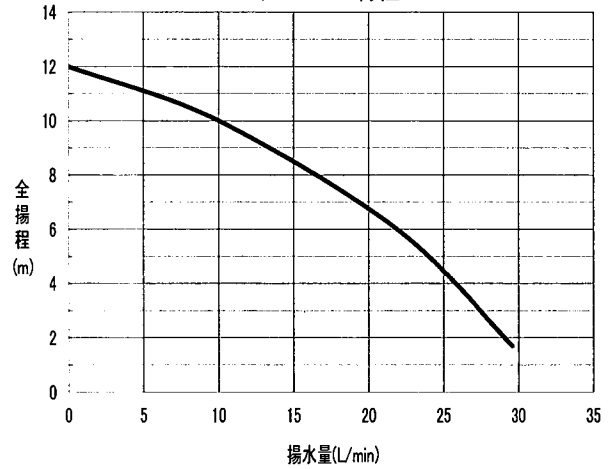
ポンプH-Q特性
