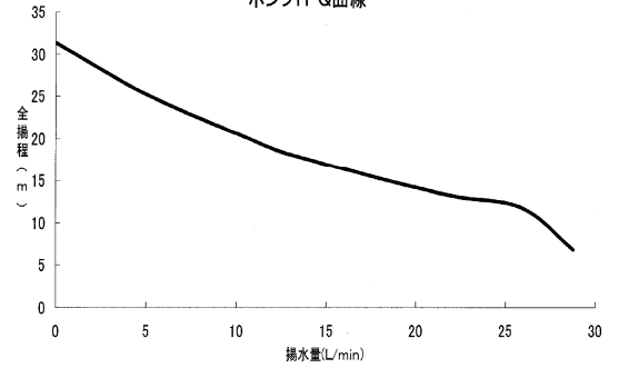
ポンプH-Q曲線
