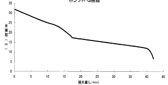
ポンプH-Q曲線
