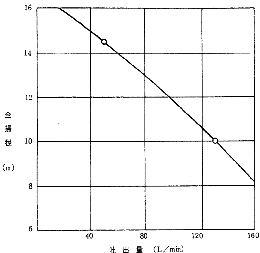
特 性 図
