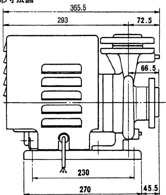
外形寸法図
