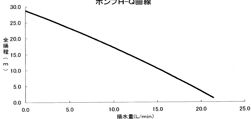
ポンプH-Q曲線
