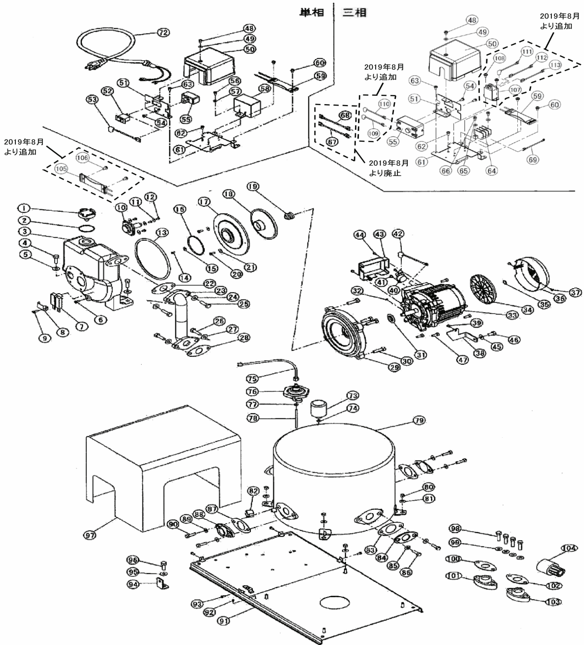
浅深用自動式ポンプ(KP-LT形400W単相、KP-LT-1形400W三相)
