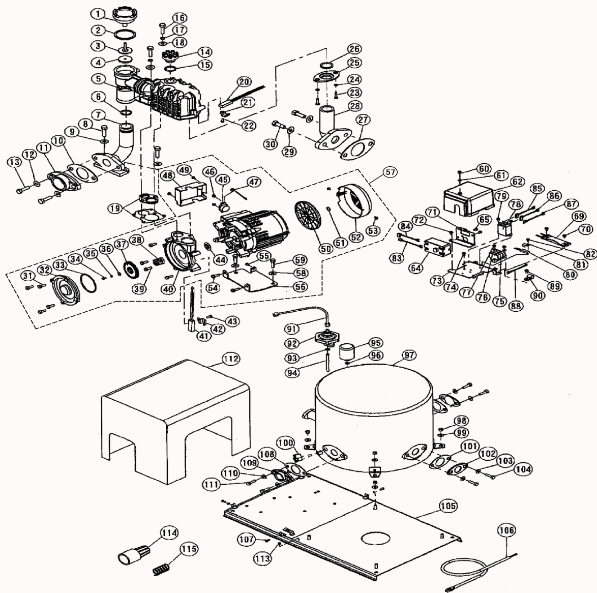
浅井戸用自動式ポンプ(WP-LT-2形 750W)
