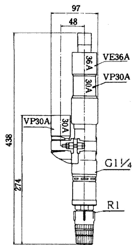
ジェット部 (別売) PG-305FS 用
