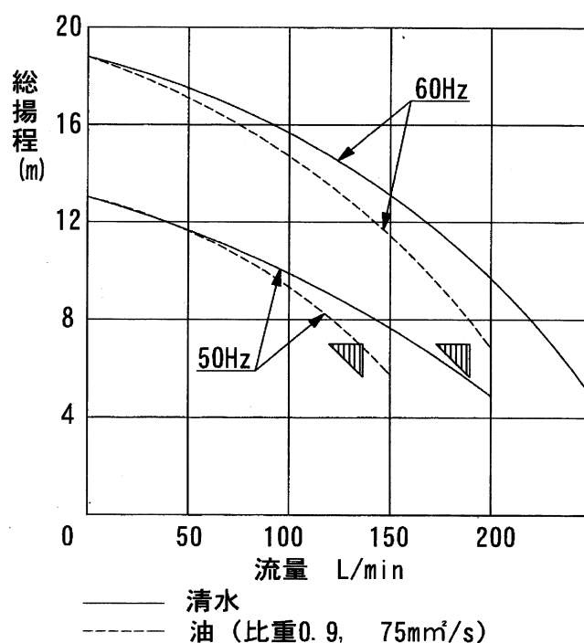
ポンプ特性
