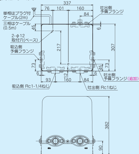
■外形寸法図 400W
