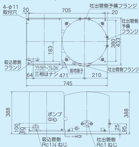
■外形寸法図 400W,750W
