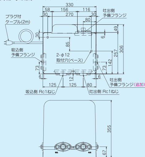
■外形寸法図 400W
