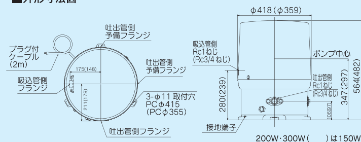
■外形寸法図
