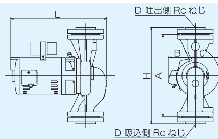
■外形寸法図 フランジ式
