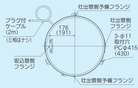
■外形寸法図 200W~750W
