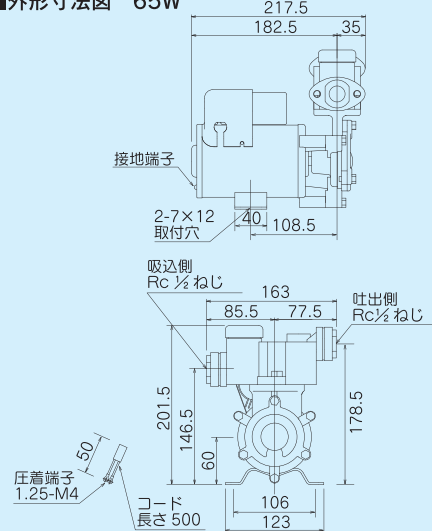
CP-155U-1/156U-1 (出力100W以上はカバー付です)
