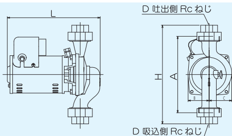
■外形寸法図 ユニオン式
