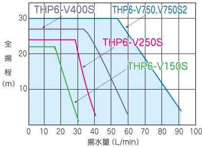
■選定図
