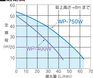
■選定図
