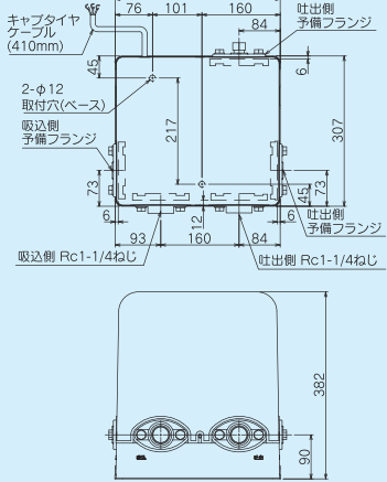
■外形寸法図 750W
