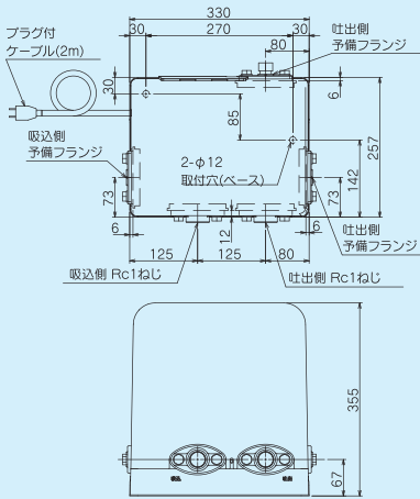
■外形寸法図 750W
