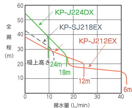
■選定図 KP-255T/256T
