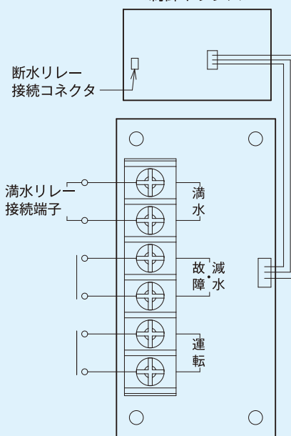
&lt;外部出力基板&gt;
