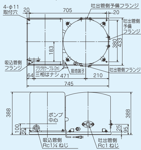
■外形寸法図 400W, 750W
