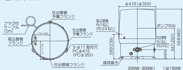
■外形寸法図
