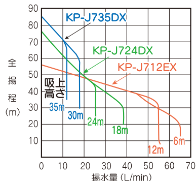
■選定図 KP-3755LT-1/3756LT-1
