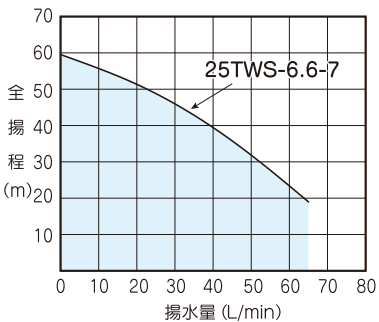
0.6kW(三相)
