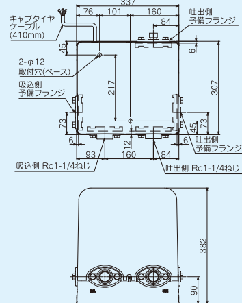
■外形寸法図 750W
